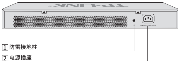
图1-4 YLS220-24G2F后面板示意图
