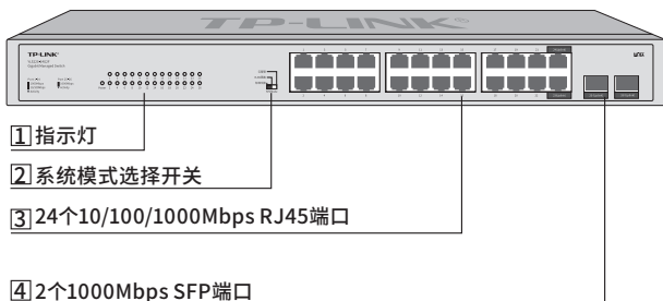
图1-2 YLS220-24G2F前面板示意图
